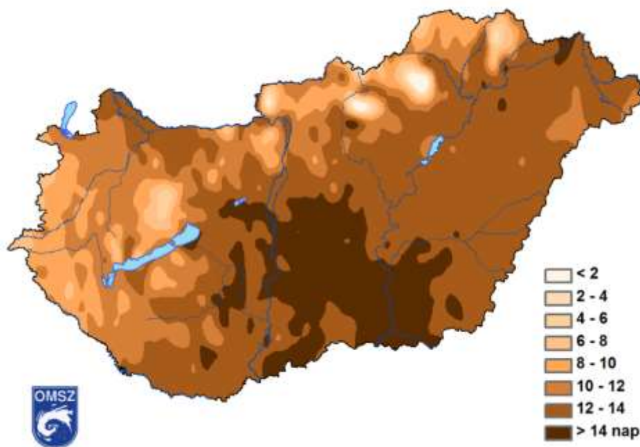
32. ábra: Hőhullámos napok száma (napi középhőmérséklet > 25^{\circ}\text{C} ) az 1981–2016-es időszakban, rácsponti trendbecslés alapján
