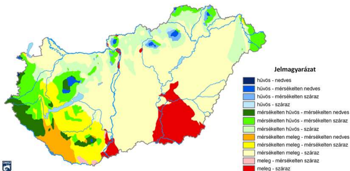
30. ábra: Magyarország éghajlati körzetei (Péczy György munkája alapján)
