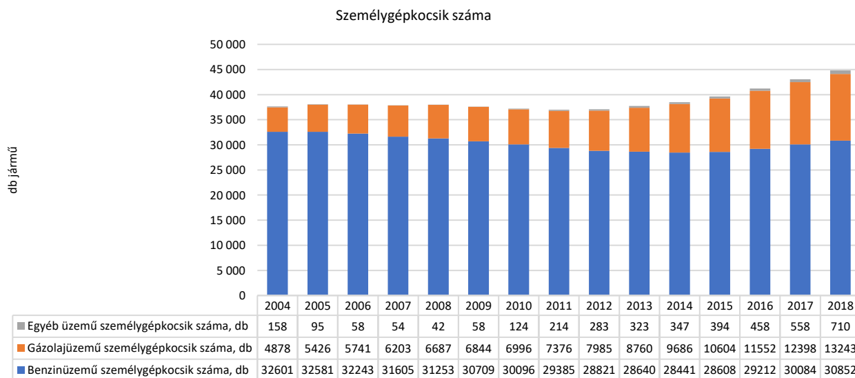
20. ábra: Gépjárművek számának alakulása Nyíregyházán 2004 és 2018 között
