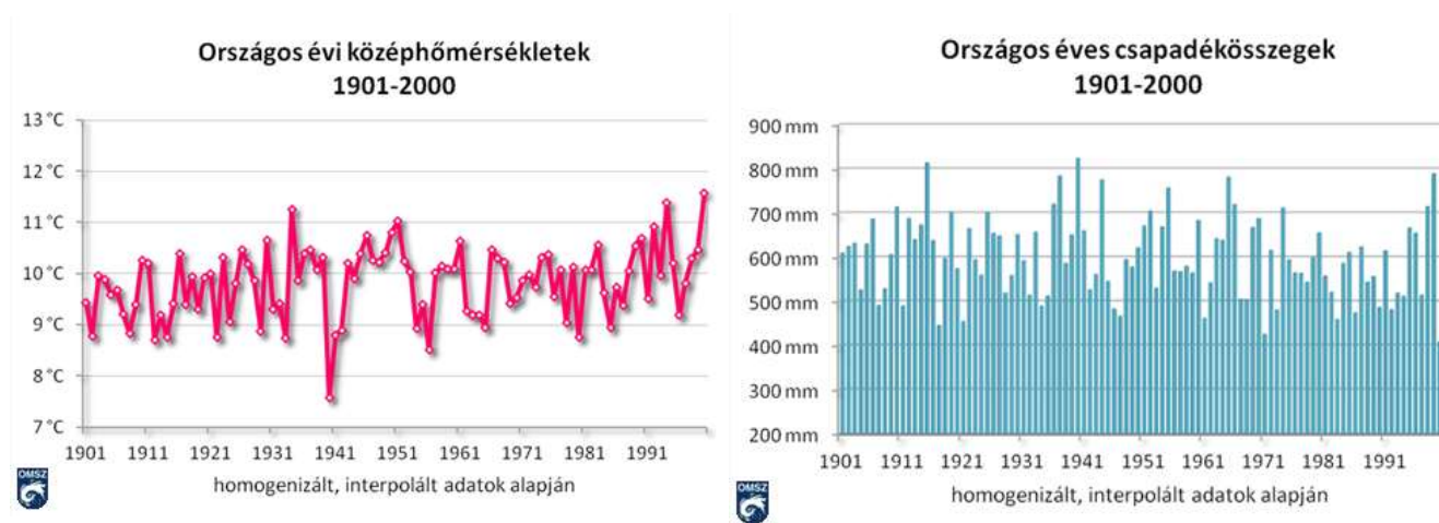
35. ábra: Országos évi középhőmérsékletek és éves csapadék összegek alakulása 1901 és 2000 között
