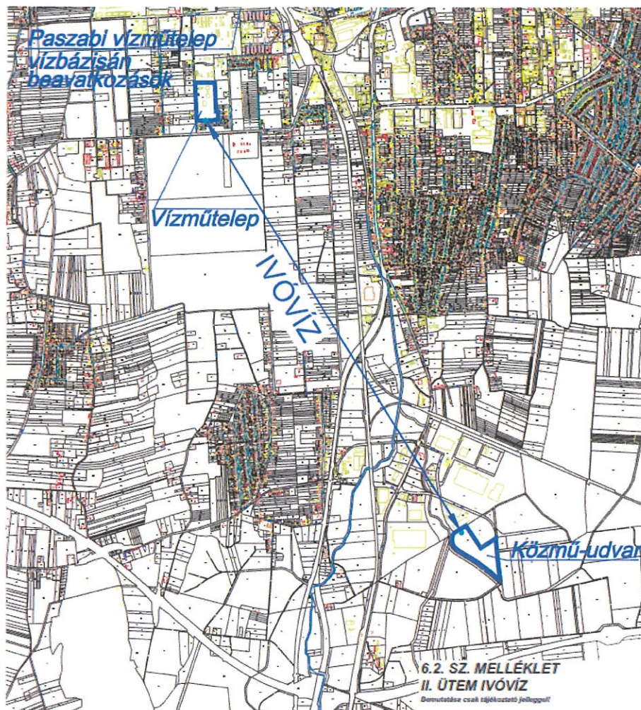
II. ütemben megvalósítandó ivóvíz hálózatfejlesztés
