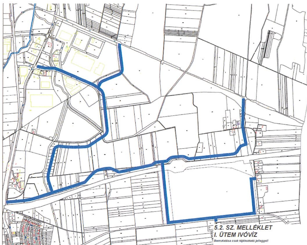
I. ütemben megvalósítandó ivóvíz hálózatfejlesztés
