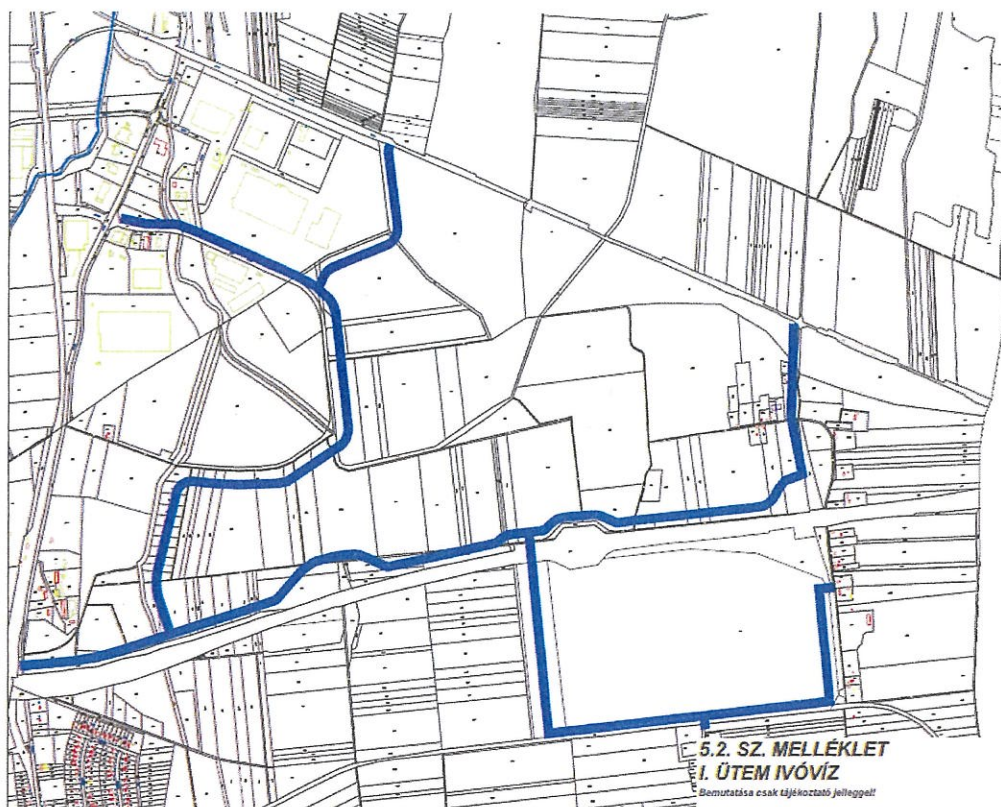
I. ütemben megvalósítandó ivóvíz hálózatfejlesztés
