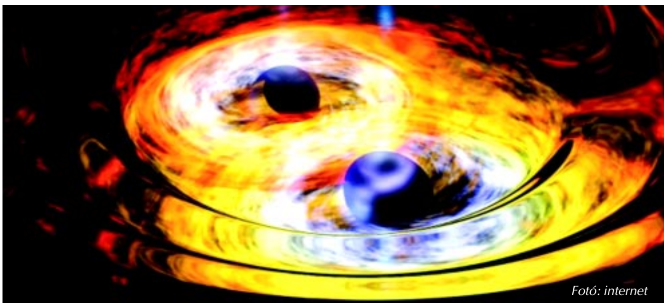
Két fekete lyuk ütközése
